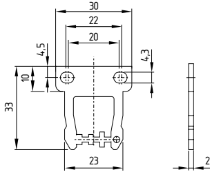
Atuador reto B1
