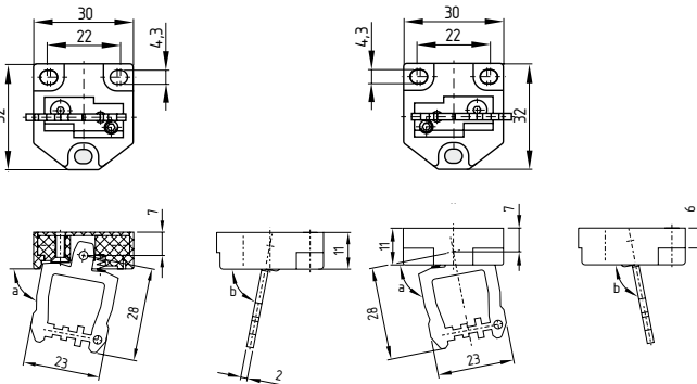
Atuador móvel B6L
