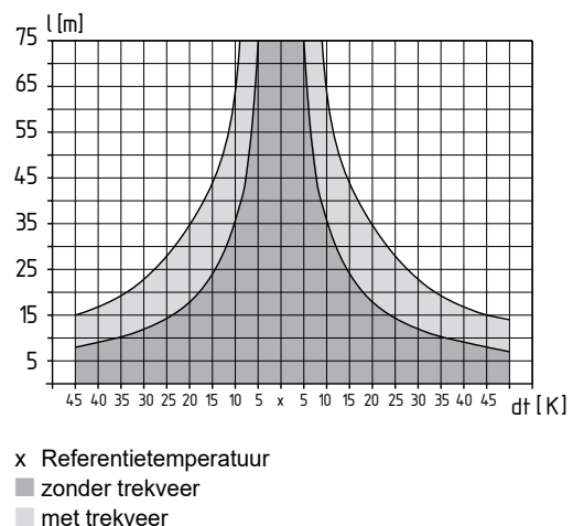
Afbeelding 4: Maximale kabellengte afhankelijk van de temperatuurverandering met of zonder trekveer
