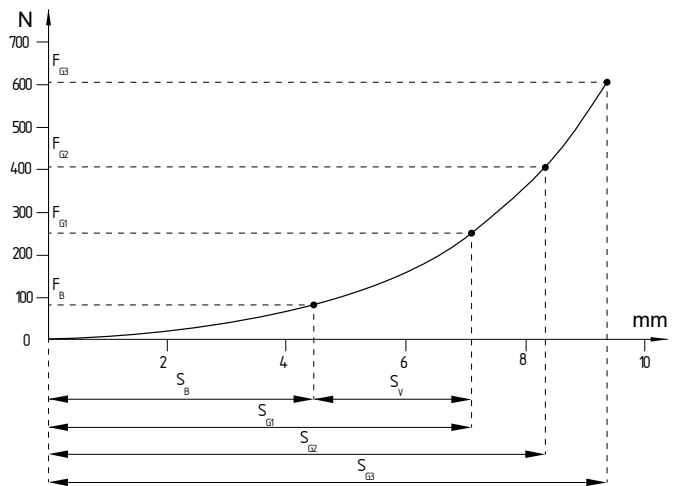
Abb. 1: Kraft-Weg-Diagramm Profil STW-SL-N-05
