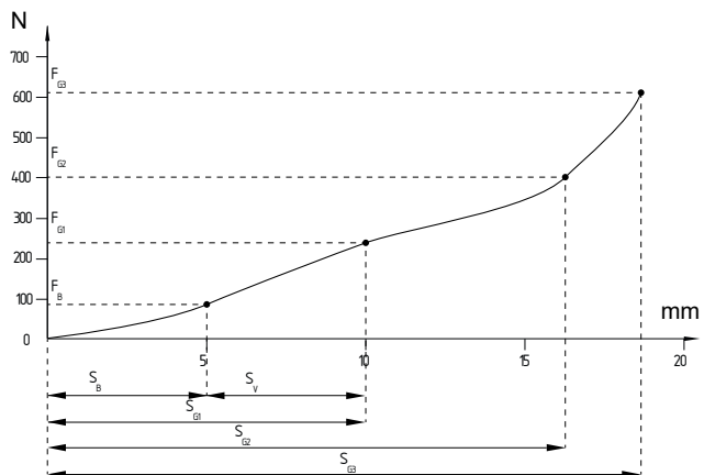
Abb. 2: Kraft-Weg-Diagramm Profil STW-SL-N-06
