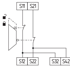
Interruptor giratorio "mode" 1, posición 2 y posición 8
