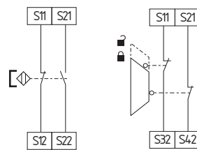
Interruptor giratorio "mode" 1, posición 3 y posición 9
