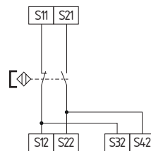
Interruptor giratorio "mode" 1, posición 1 y posición 7
