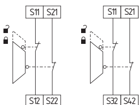
Interruptor giratorio "mode" 1, posición 2 y posición 8
