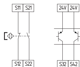
Interruptor giratorio "mode" 1, posición 4 y posición 10
