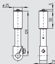
Bandscheefloophefboom 243
