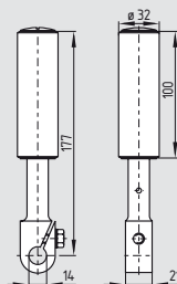
Bandscheefloophefboom 1224
