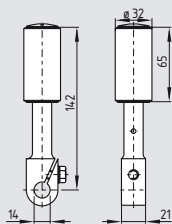
Bandscheefloophefboom 966
