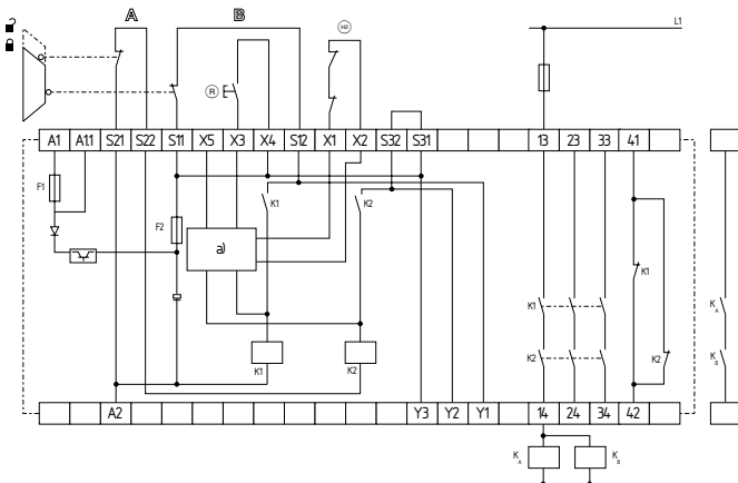
Abb. 5 a) Ansteuerung
