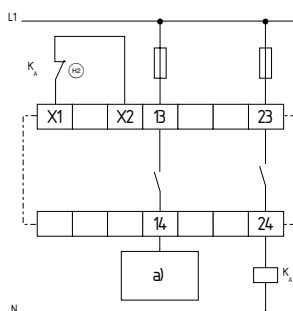
Abb. 19 a) Reglerfreigabe
