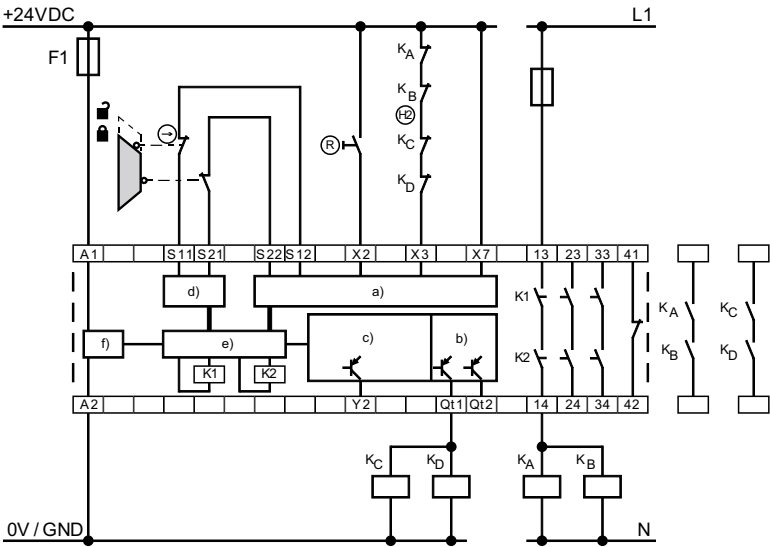
SRB-E-322STの配線例
