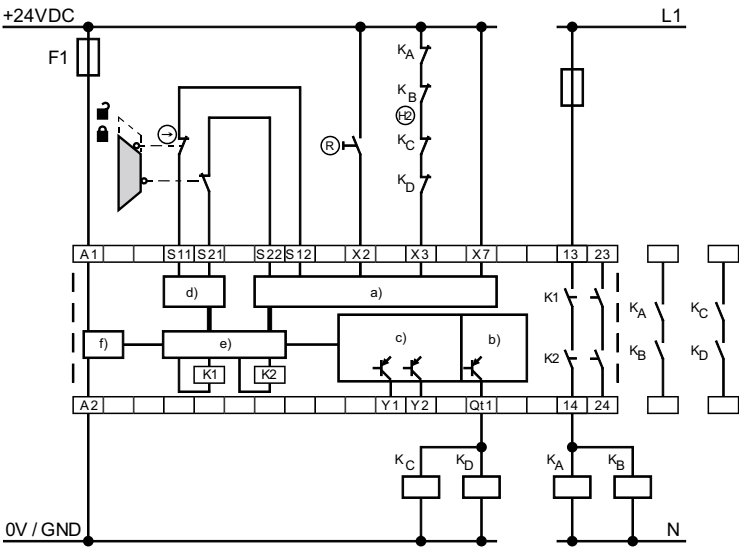
SRB-E-212STの配線例
