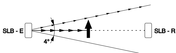
Rys. 1b: Funkcja bezpieczeństwa zagwarantowana
