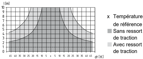
Image 4: Longueur maximale du câble en fonction de la température avec ou sans ressort de traction
