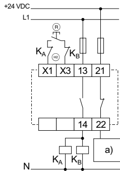
Fig. 18 a) Bloc logique Ⓡ = Bouton de réarmement Ⓜ = Boucle de retour
